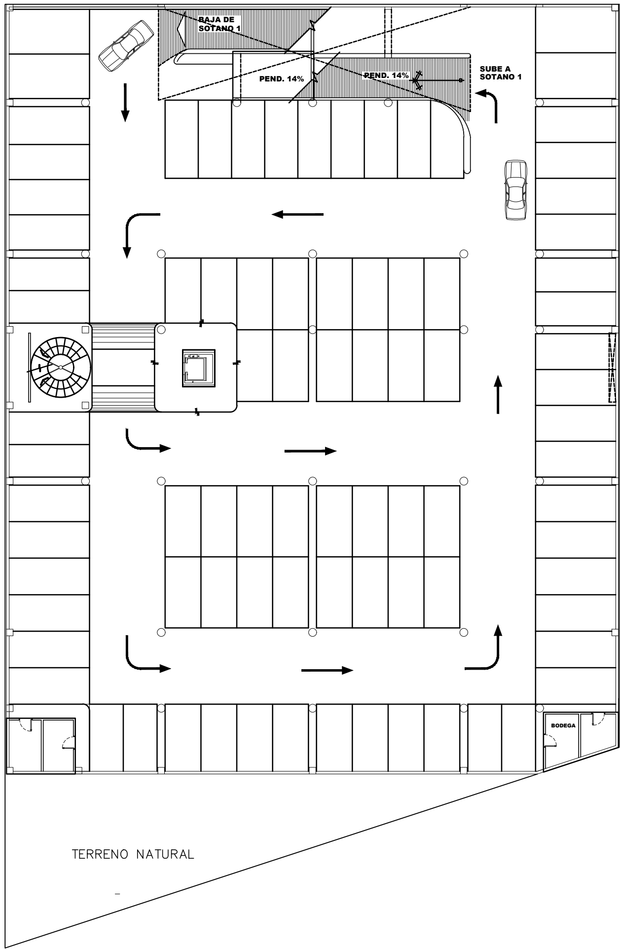
PLANTA SOTANO 2
